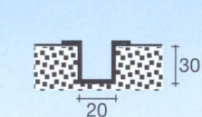
Guida inferiore incassata per passaggio carrello
