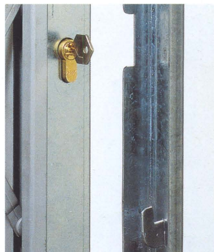
SERRATURA A CILINDRO EUROPEO
